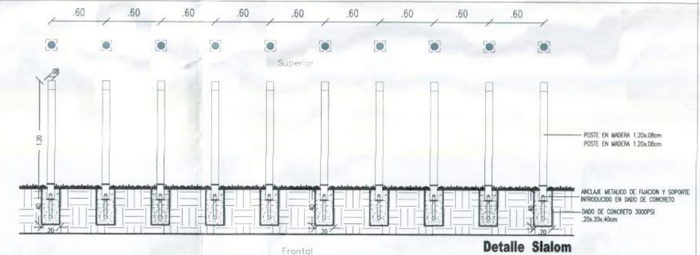
Detalle Slalom Escala 1:25
