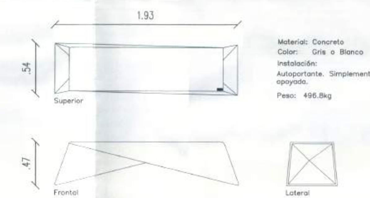
Detalle banca en concreto referencia: mc konkretus Escala 1:25
