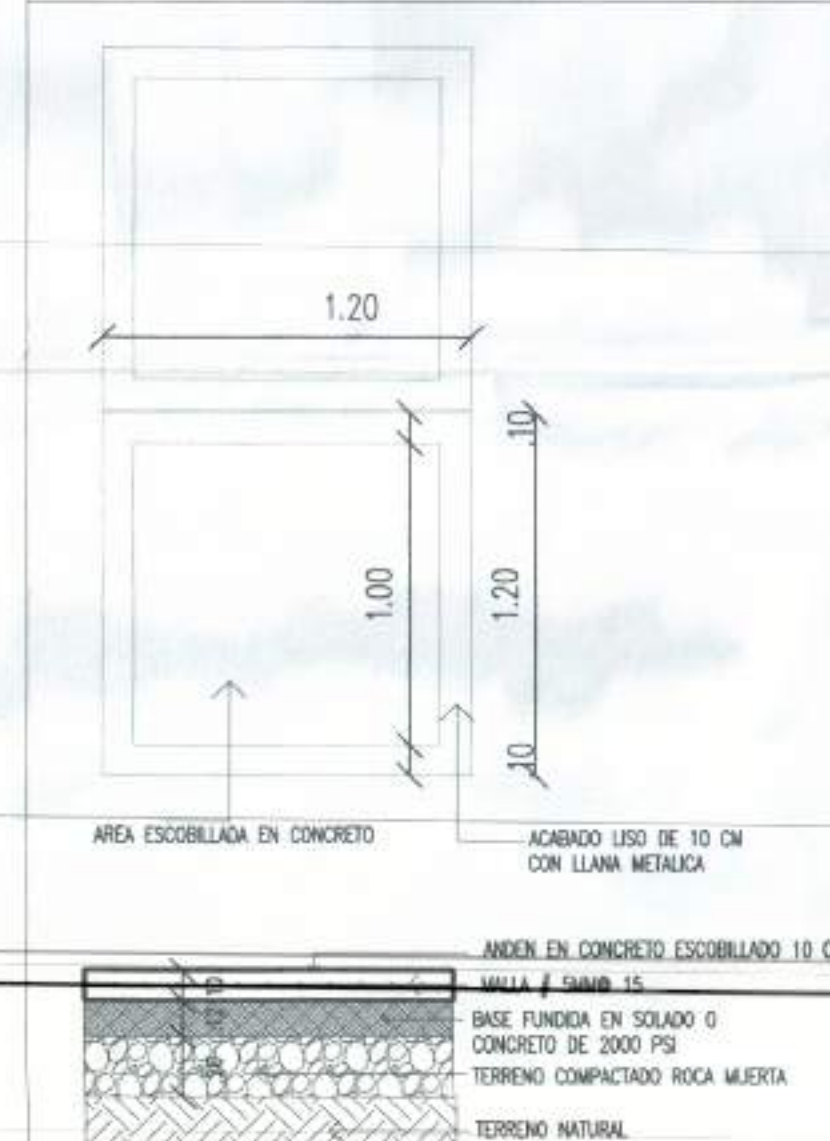
Detalle andén en concreto escobillado Escala 1:25
