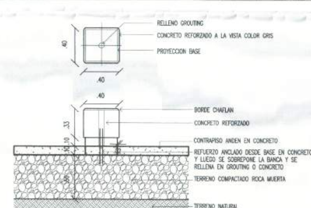
Detalle banca tipo cubo Escala 1:25
