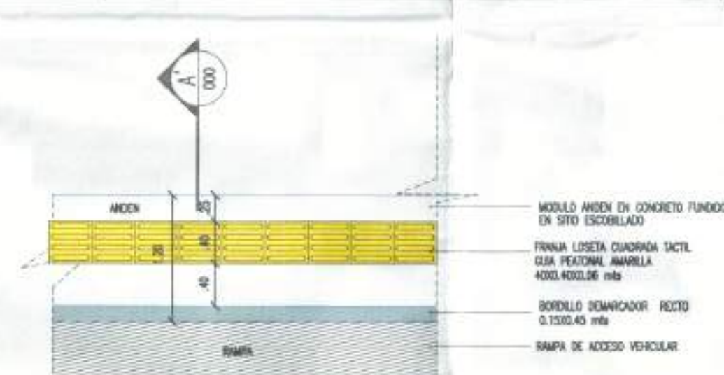
Detalle anden peatonal y rampa escala 1:50
