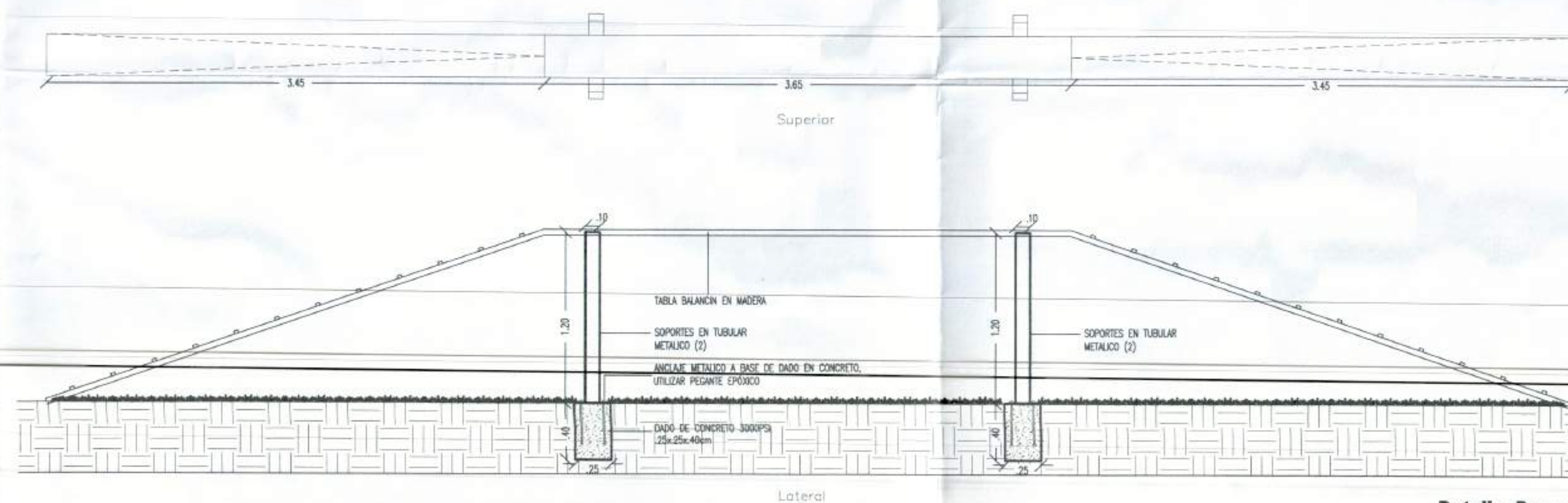
Detalle Pasarela Escala 1:25
