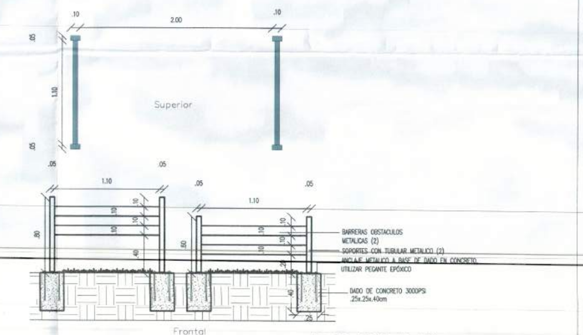
Detalle Valla Metalica Escala 1:25
