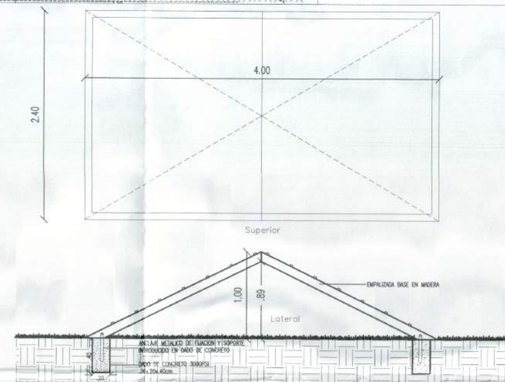
Detalle Empalizada Escala 1:25
