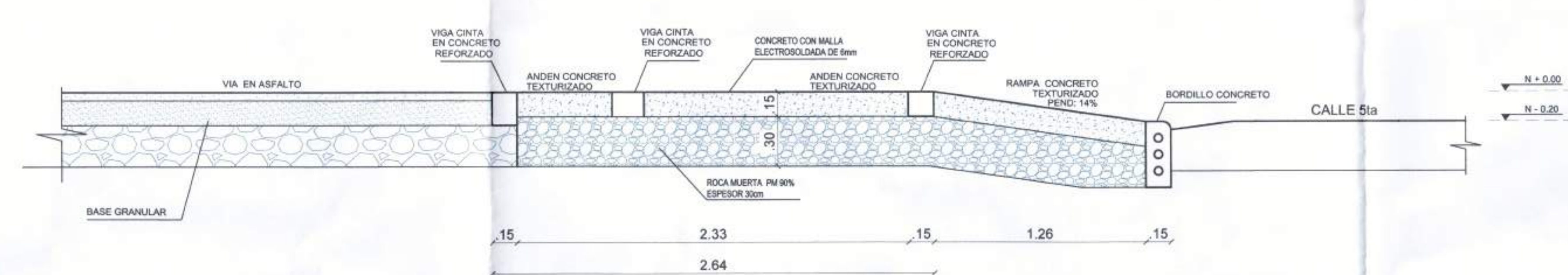
CORTE A - A' ESC : 1 : 20
