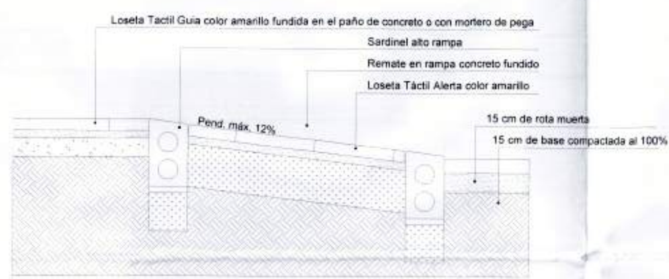
DETALLE RAMPA ESC. 1:20
