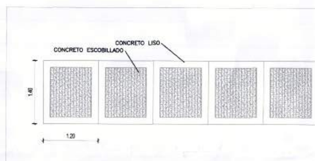
DETALLE PISO SENDERO ESC. 1:50
