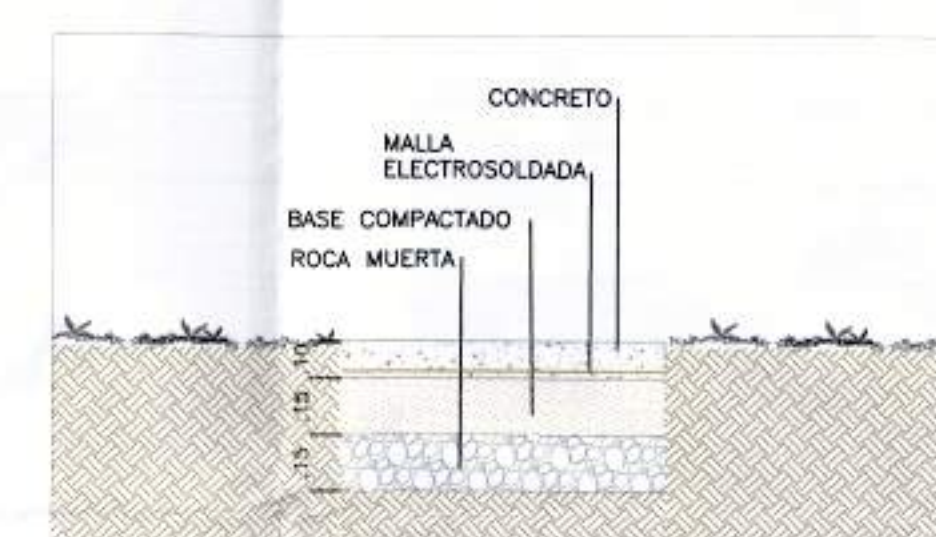
DETALLE CONSTRUCTIVO PLAZOLETA ESC. 1:20
