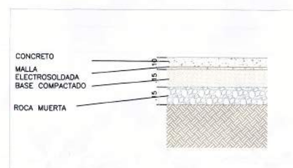
DETALLE CONSTRUCTIVO SENDERO ESC. 1:20
