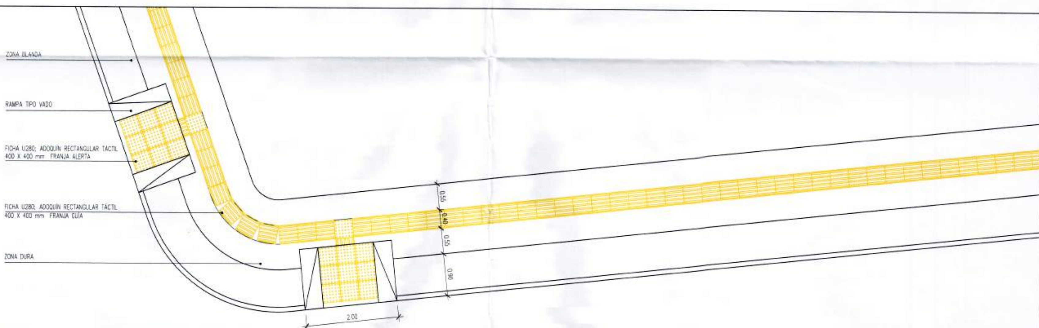
SANDÉN + RAMPA ESC 1:20
