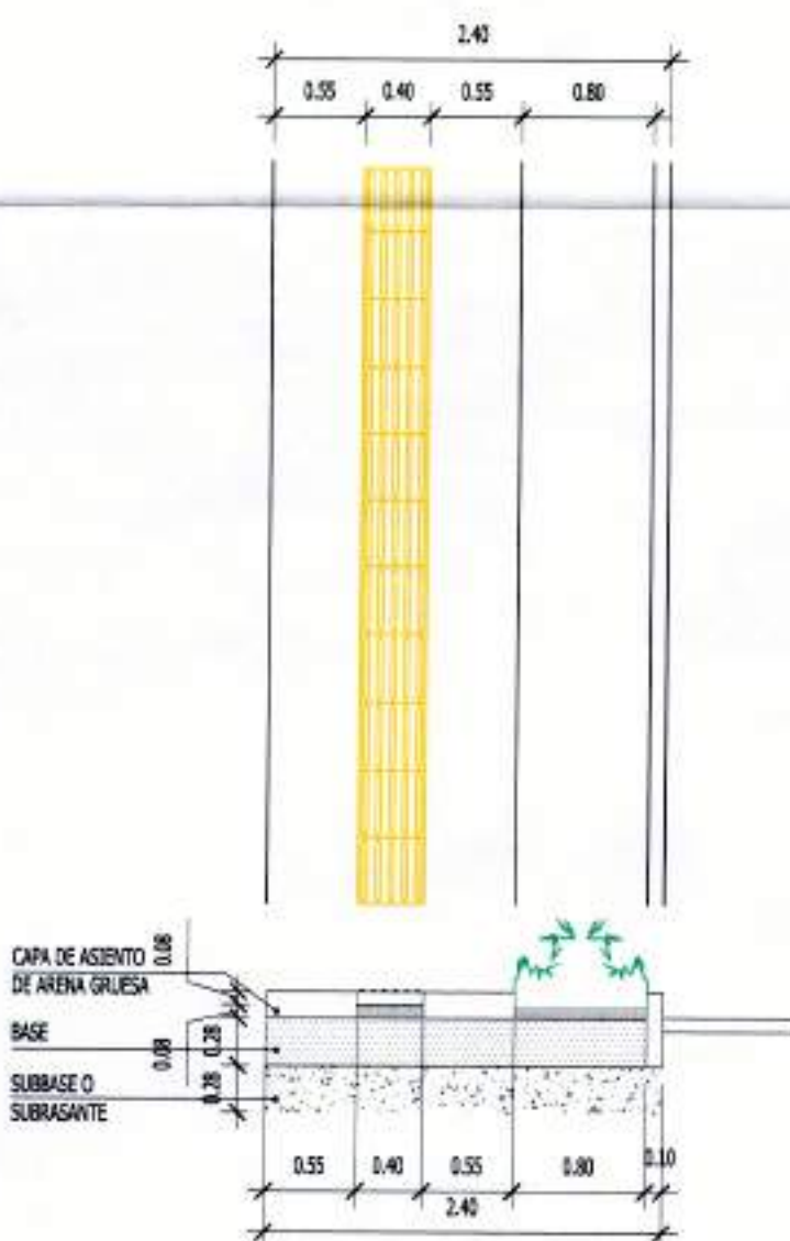
SENDERO PEATONAL ESC 1:50
