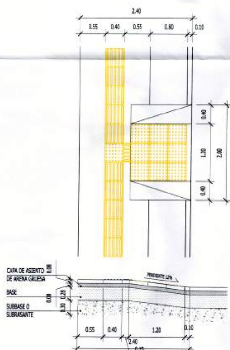
RAMPA TIPO VADO ESC 1:50
