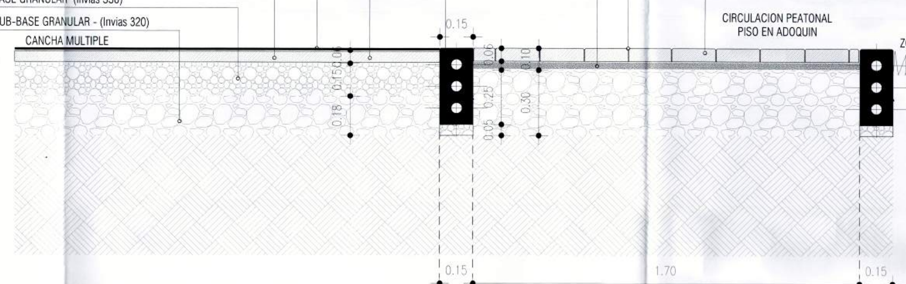
DETALLE ACABADO PISO CIRCULACION PEATONAL Y CNCHA MULTIPLE
