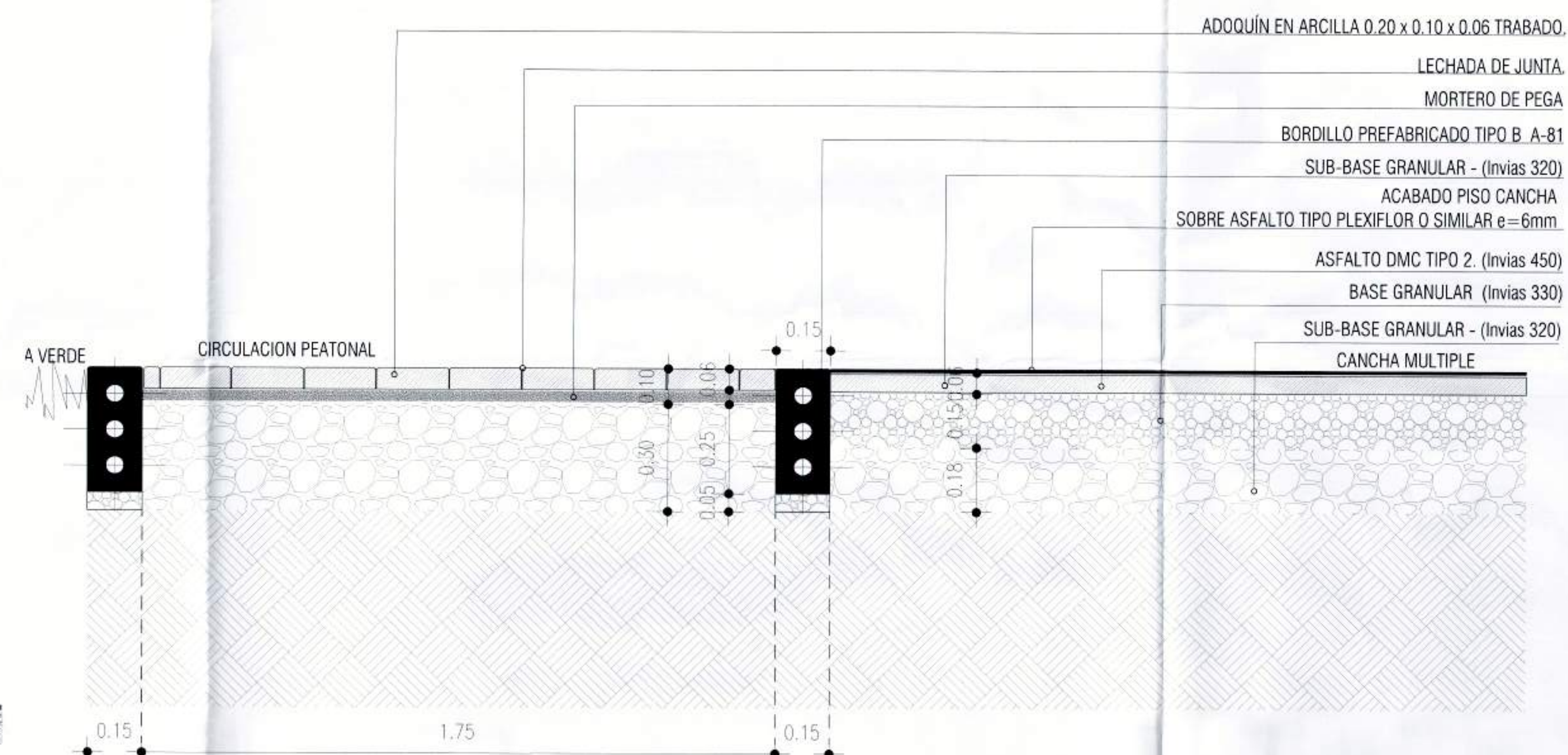
DETALLE ACABADO PISO CIRCULACION PEATONAL Y CNCHA MULTIPLE ESCALA 1: 10
