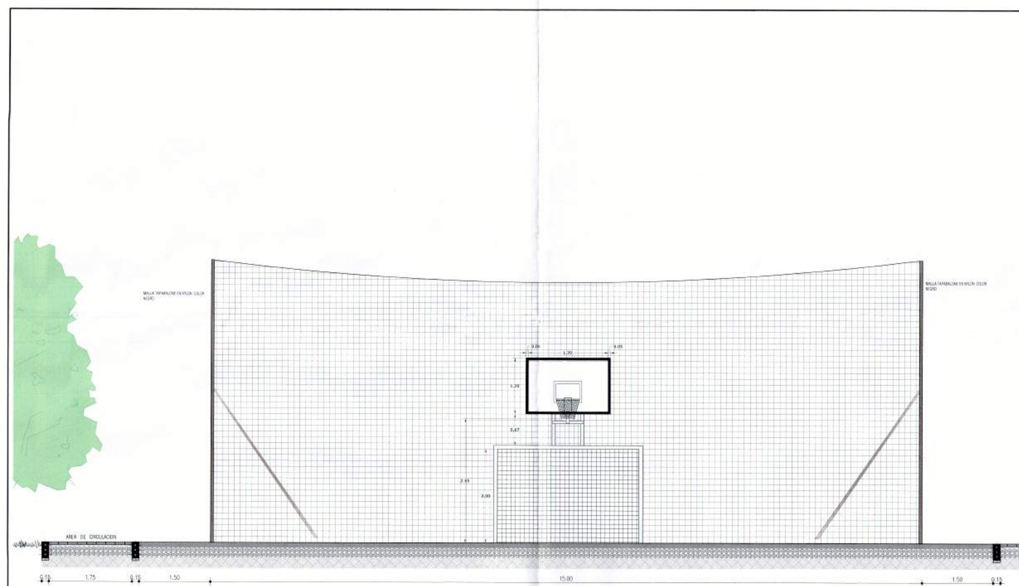
CORTE TRANSVERSAL B B' ESCALA 1: 50
