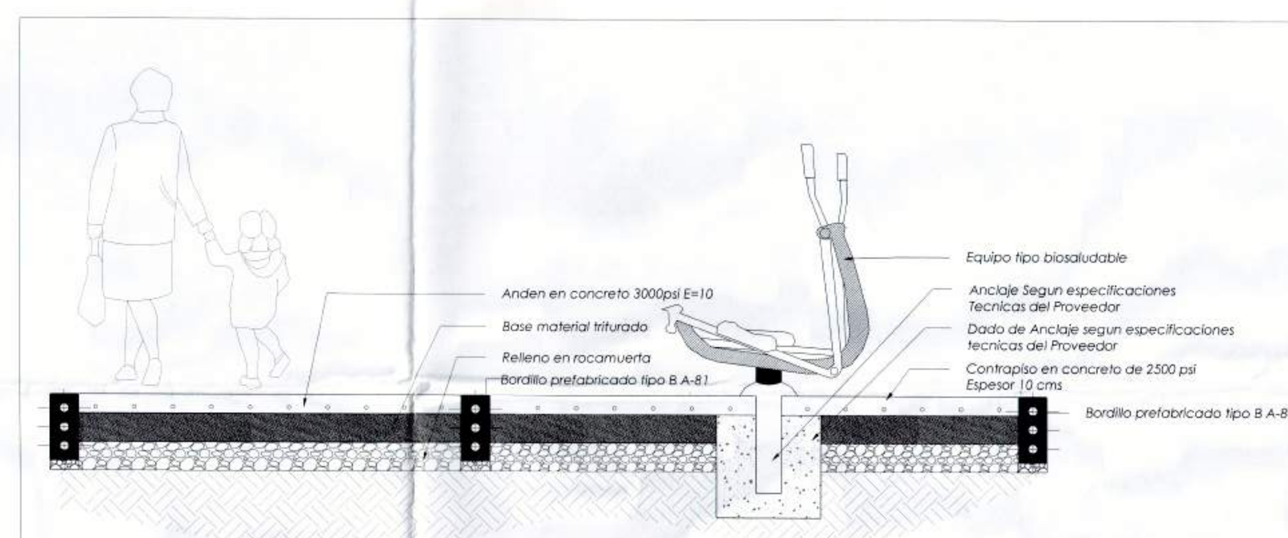
SECCION TIPO CIRCUITO BIOSALUDABLE ESC 1 : 20
