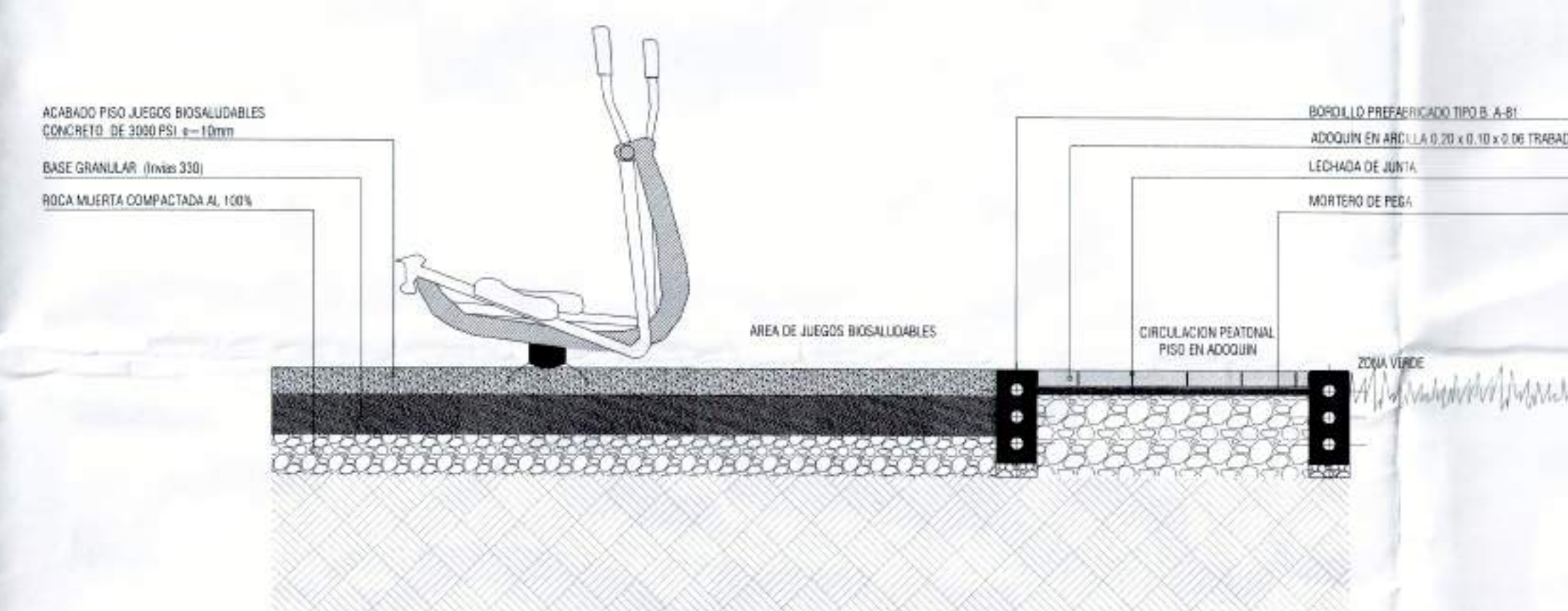
DETALLE ACABADO PISO CIRCULACION Y JUEGOS BIOSALUDABLES
