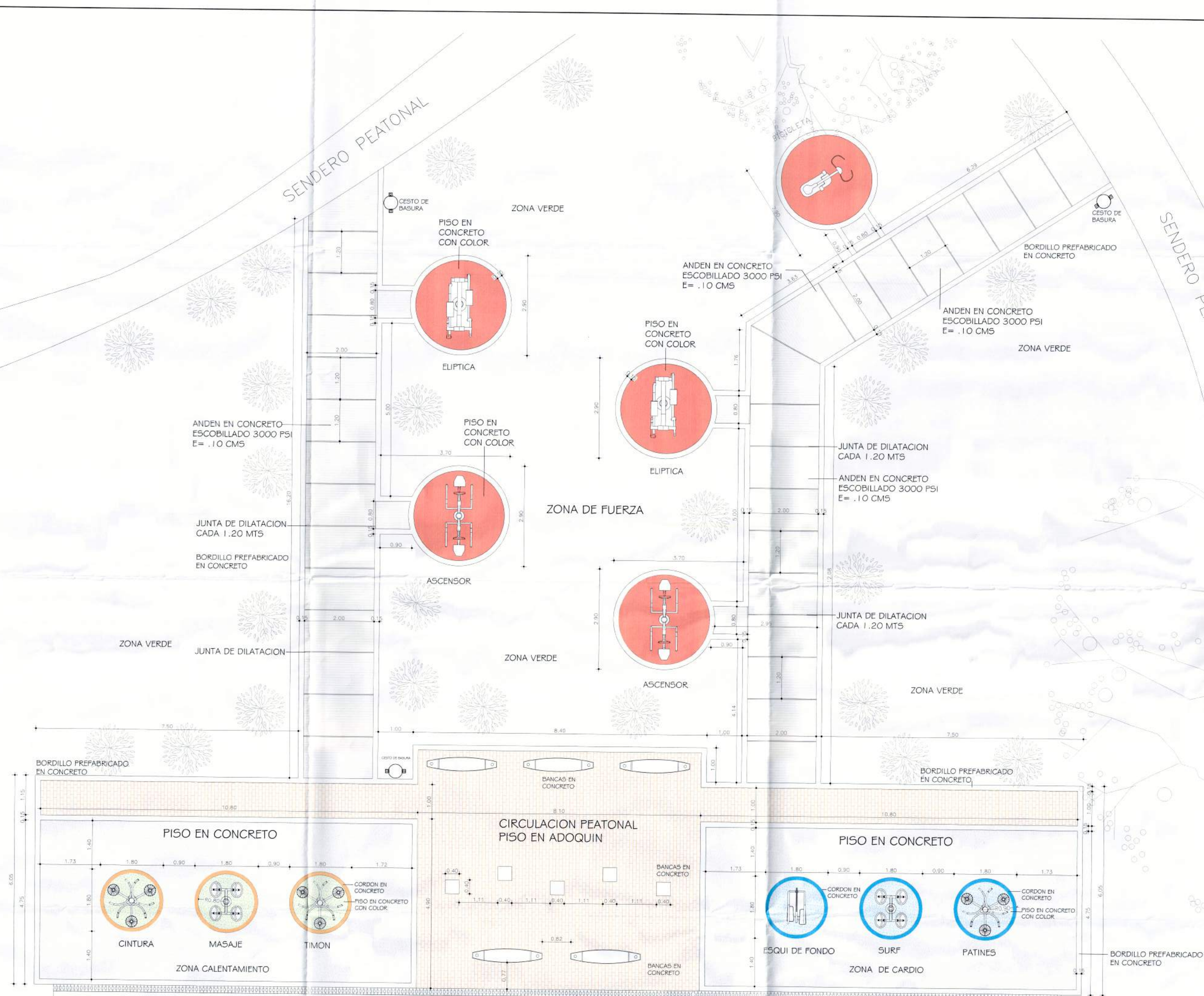
PLANTA CIRCUITO BIOSALUDABLE ESCALA 1: 50
