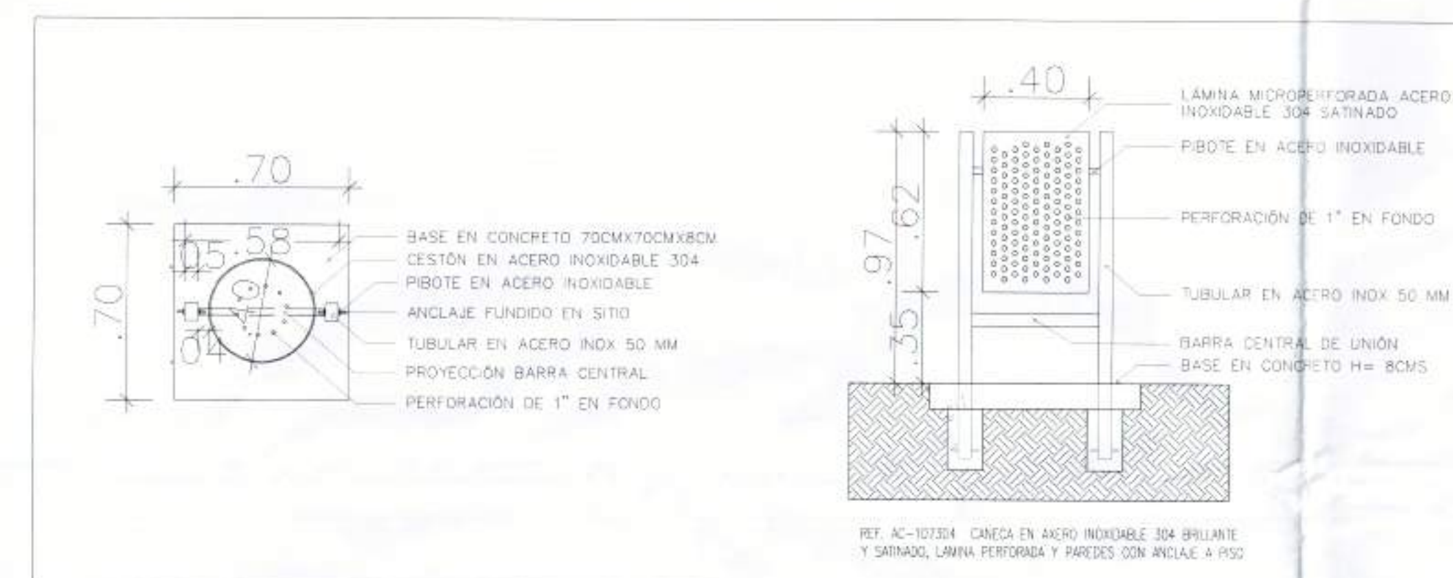
DETALLE CESTO DE BASURA EN ACERO INOXIDABLE ESC 1 : 20
