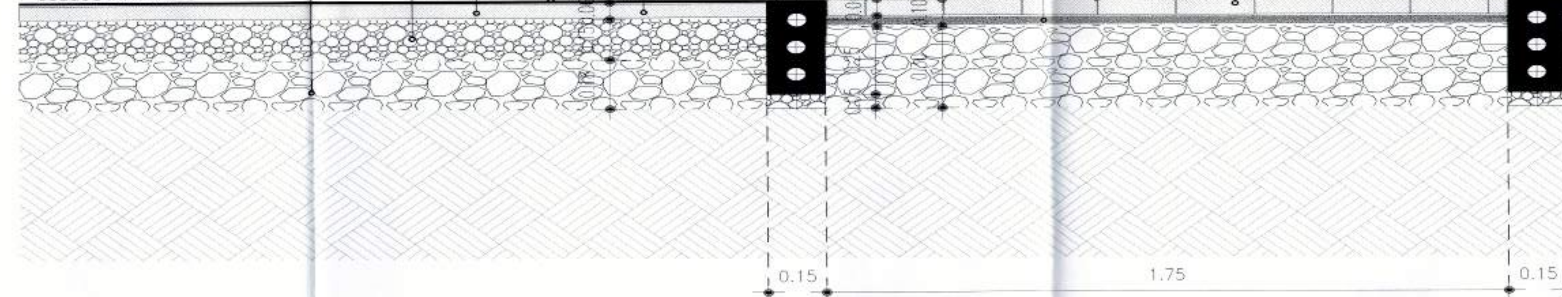
DETALLE ACABADO PISO CIRCULACION JUEGOS INFANTILES ESCALA 1 : 10
