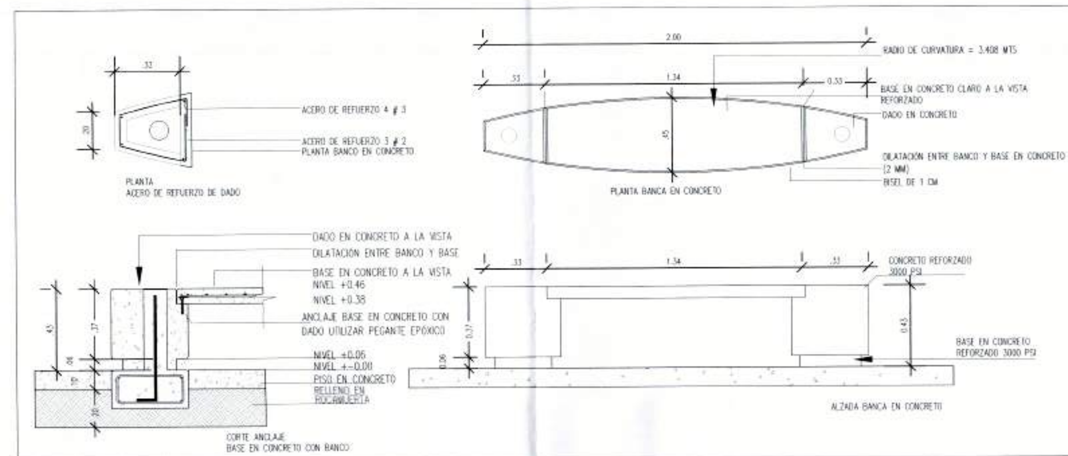
DETALLE BANCA EN CONCRETO ESC 1 : 20
