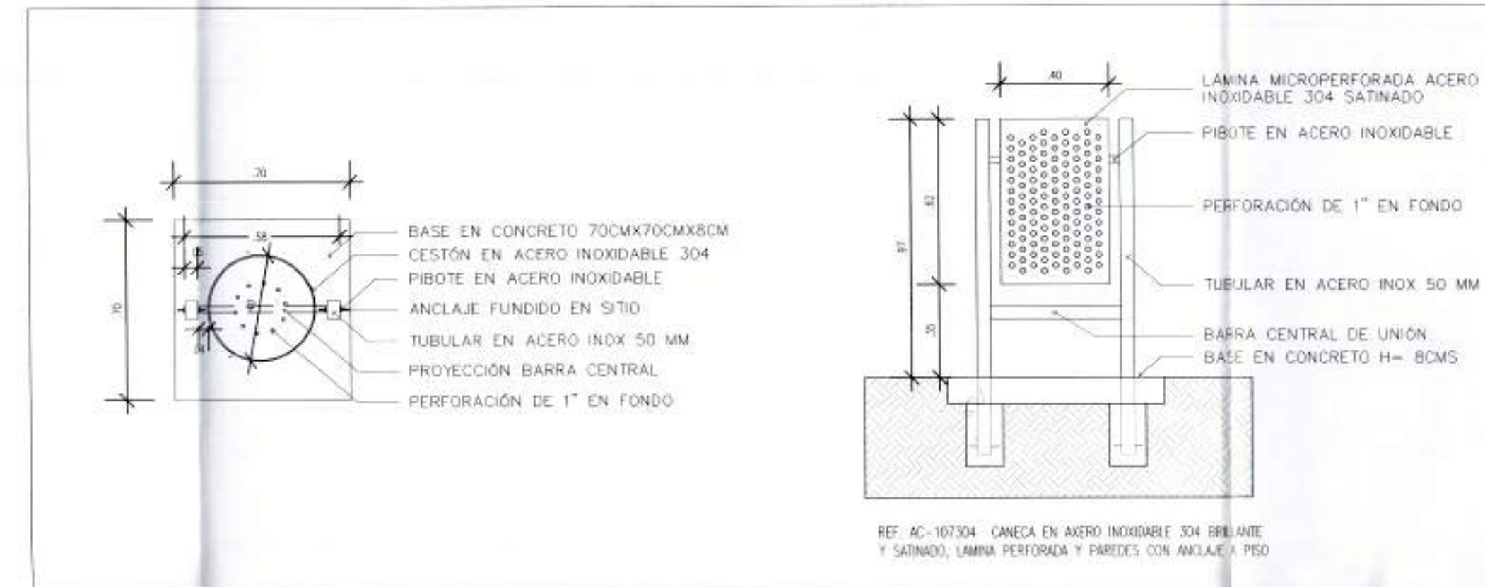
DETALLE CESTO DE BASURA EN ACERO INOXIDABLE ESC 1 : 20
