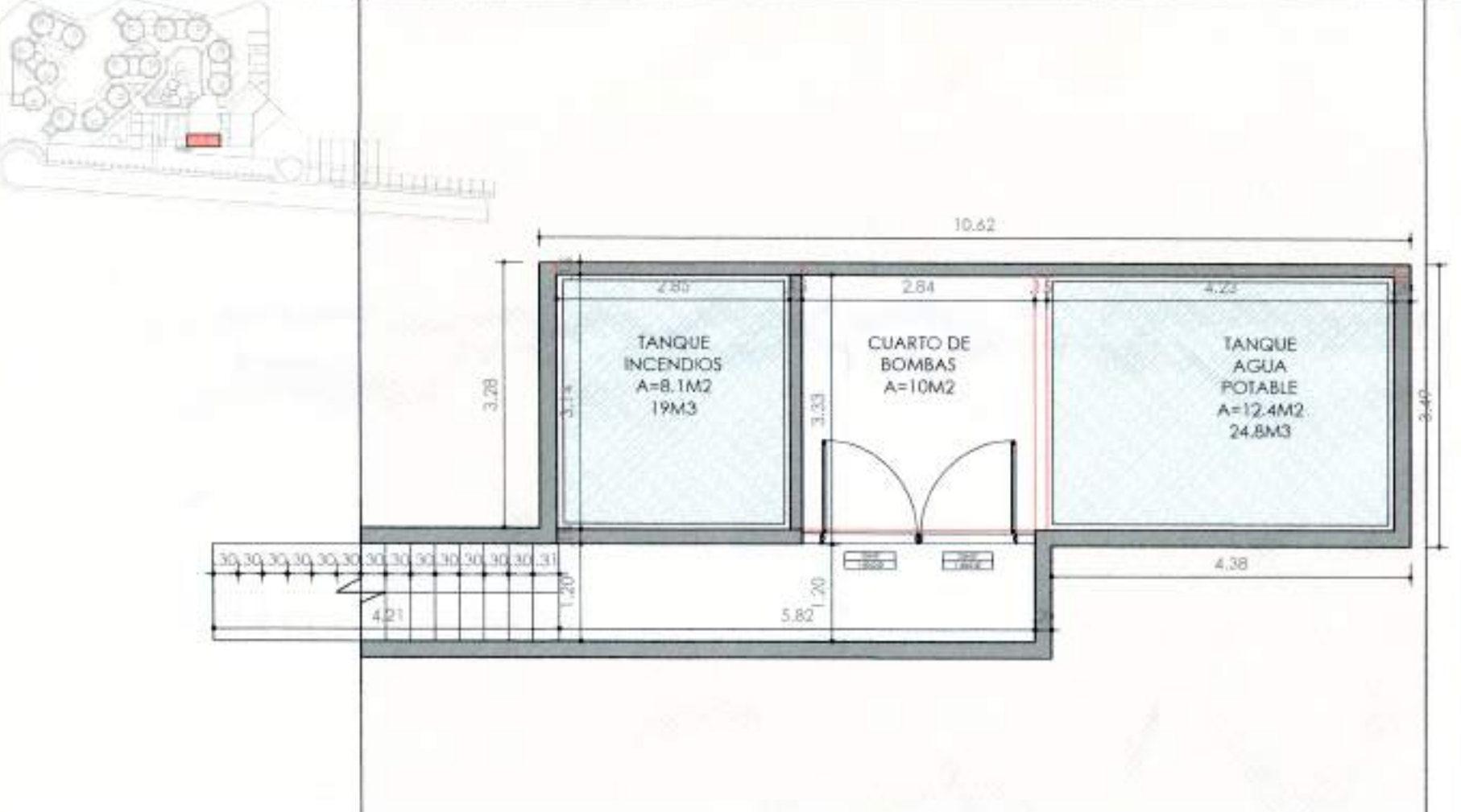
PLANTA SOTANO ESCALA 1 : 75
