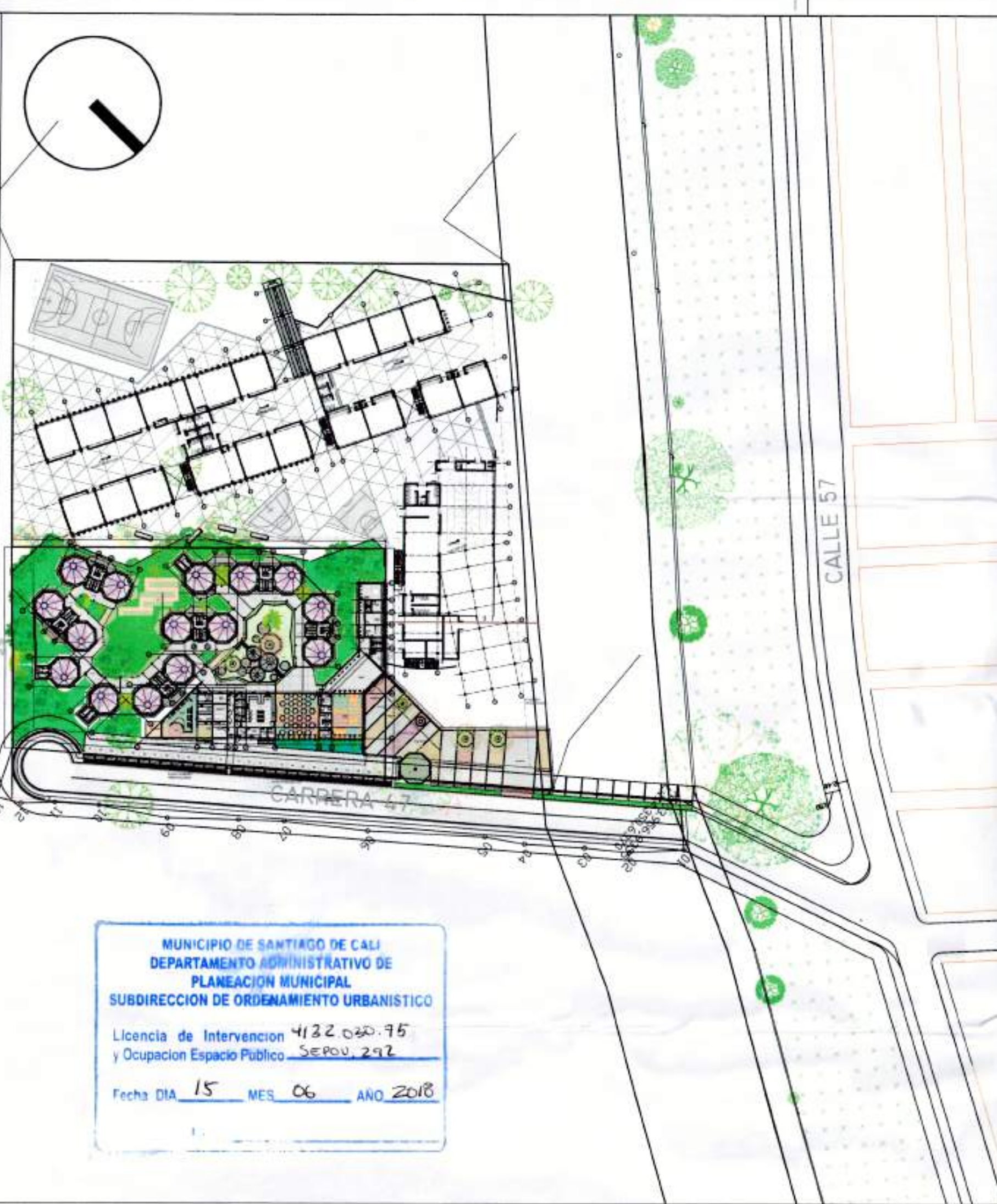
PLANTA LOCALIZACION ESCALA 1 : 1000
