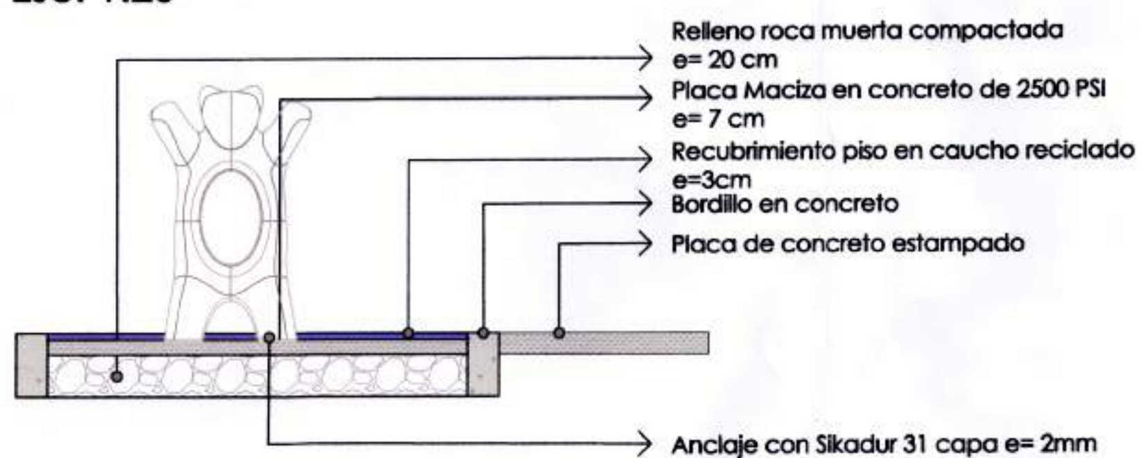
DETALLE OSO EN CONCRETO Esc. 1:25
