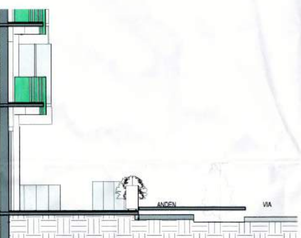
Tipo: SECCION EP1 Escala: 1 : 100
