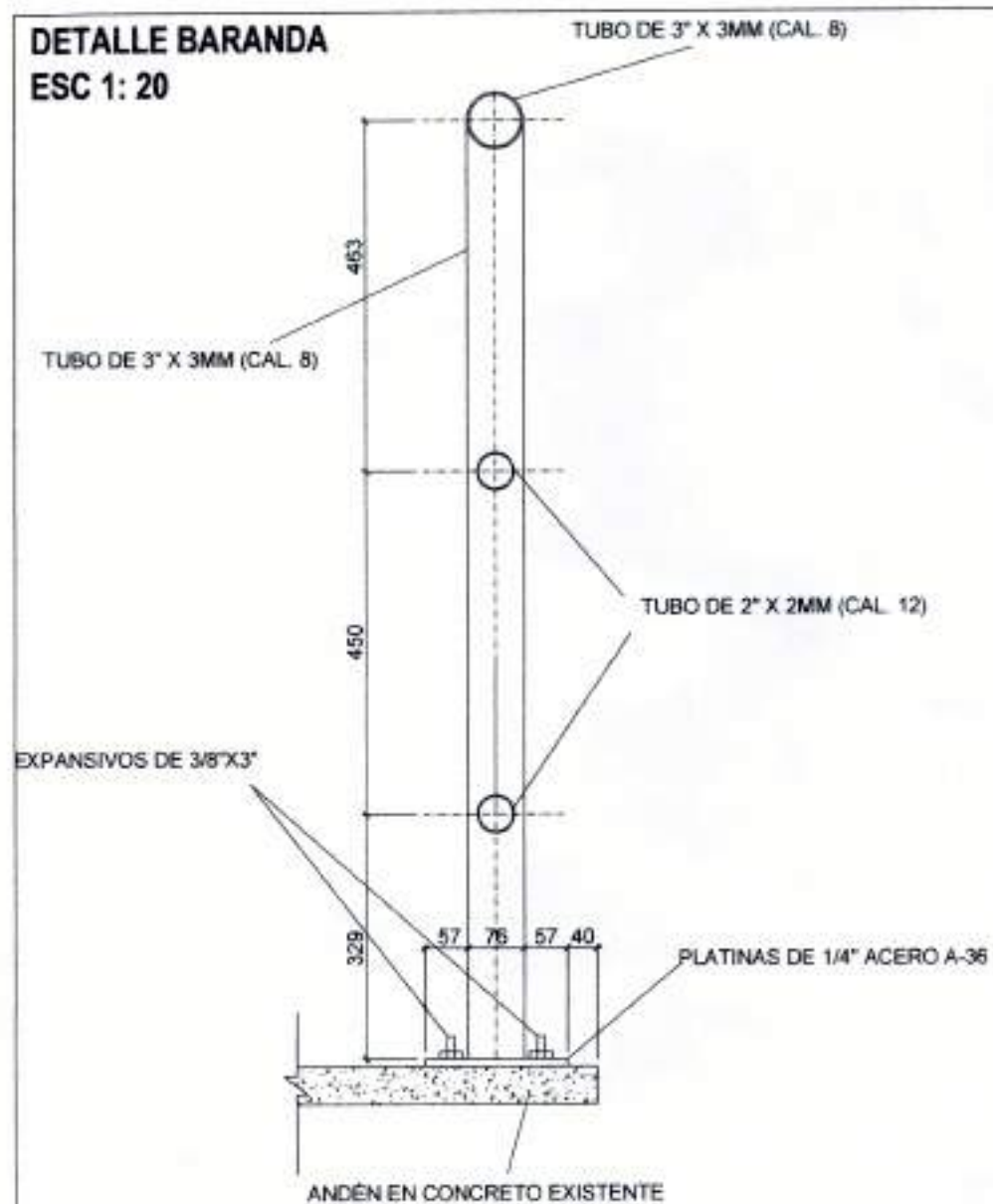
DETALLE DE BARANDAS DE PROTECCIÓN MEDIDAS EN MM
