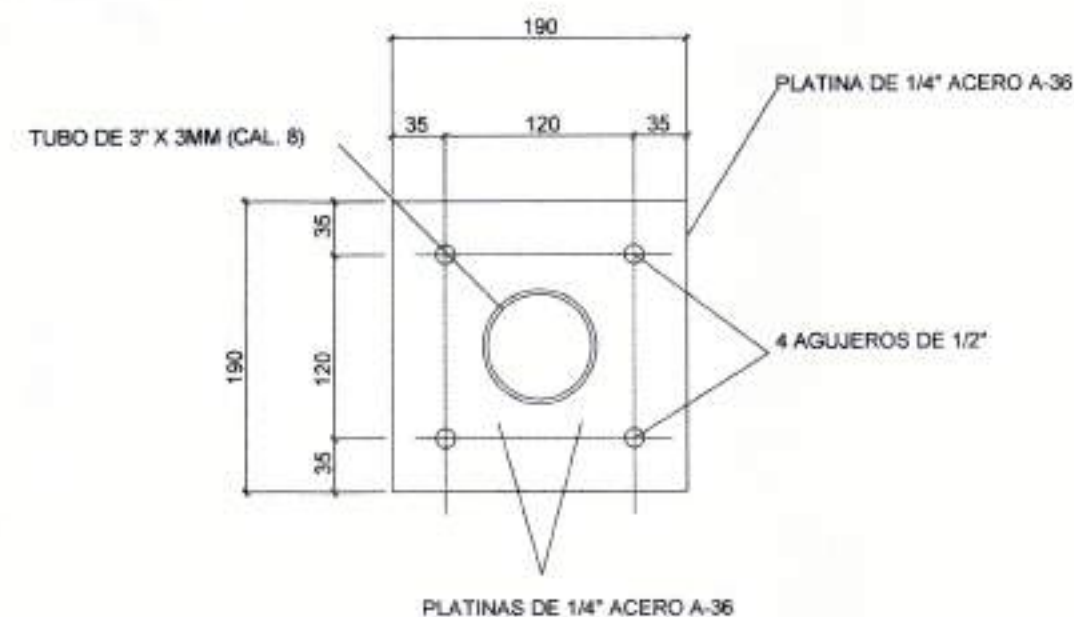
DETALLE PLATINAS DE APOYO MEDIDAS EN MM
