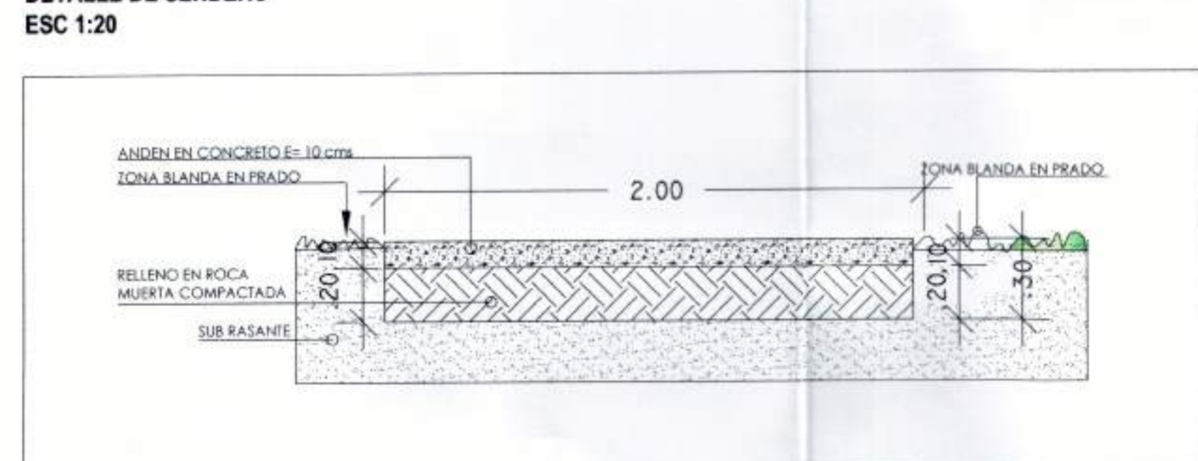
DETALLE DE SENDERO ESC 1:20
