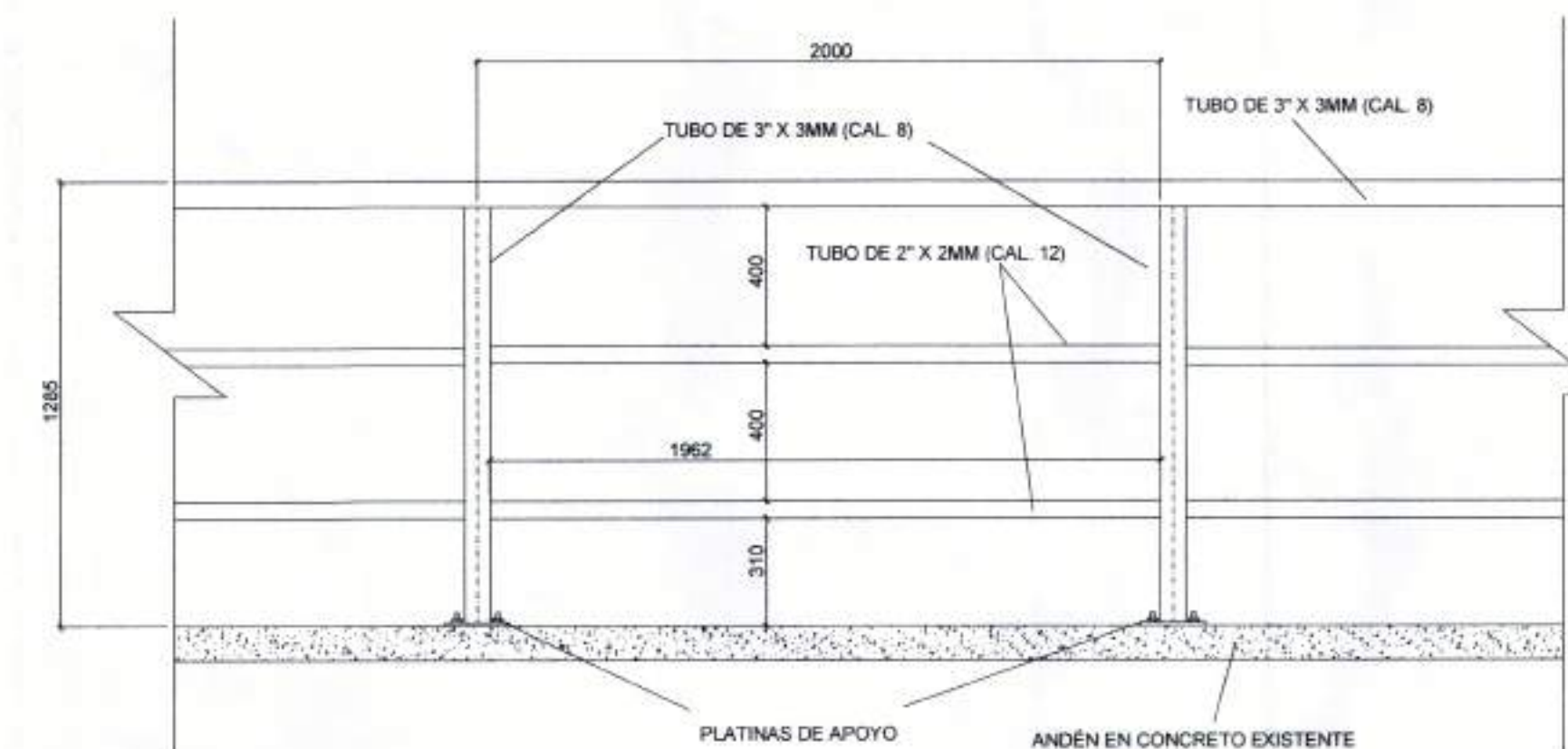
DETALLE DE BARANDAS DE PROTECCIÓN MEDIDAS EN MM
