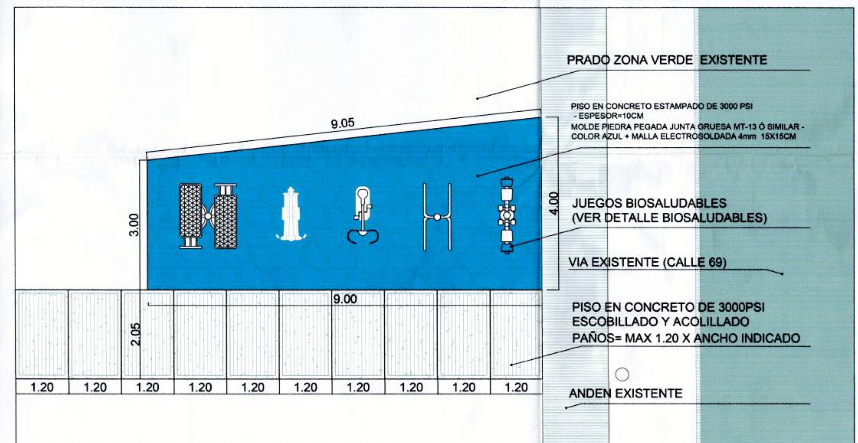
DETALLE ZONA BIOSALUDABLES ESC 1:50
