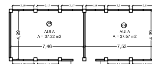
PLANTA SEGUNDO PISO
