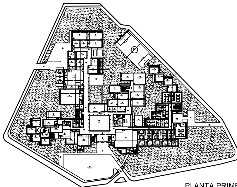
PLANTA PRIMER PISO
