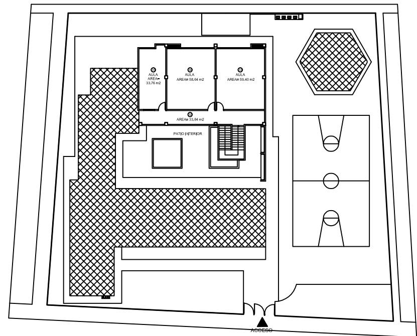
PLANTA SEGUNDO PISO
