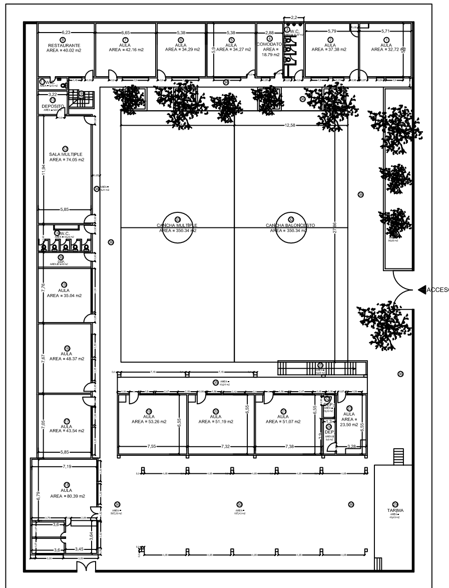
PLANTA PRIMER PISO
