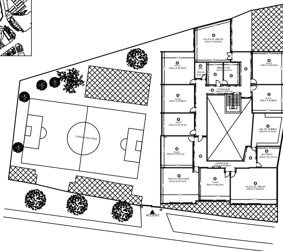
PLANTA SEGUNDO PISO
