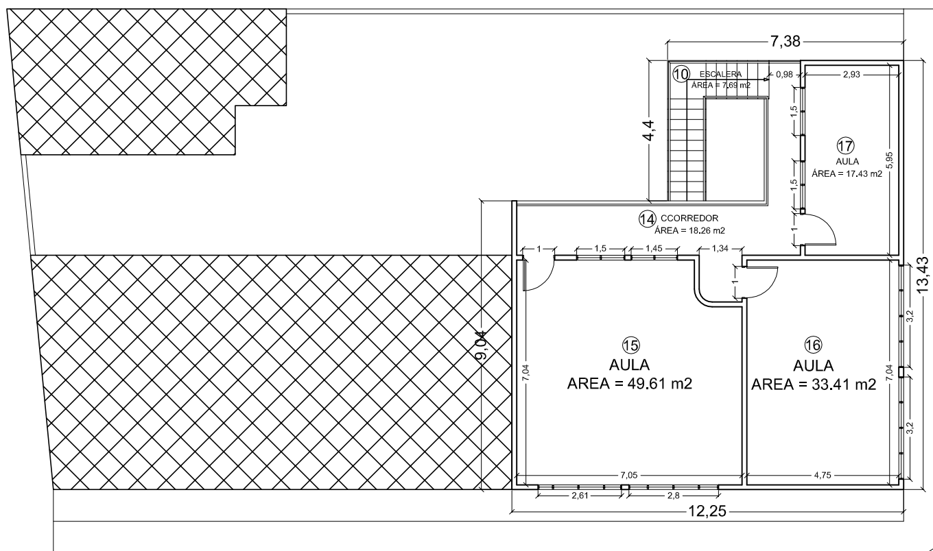
PLANTA SEGUNDO PISO
