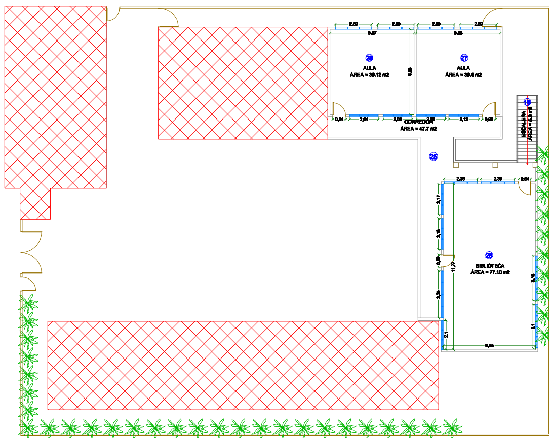
PLANTA SEGUNDO PISO
