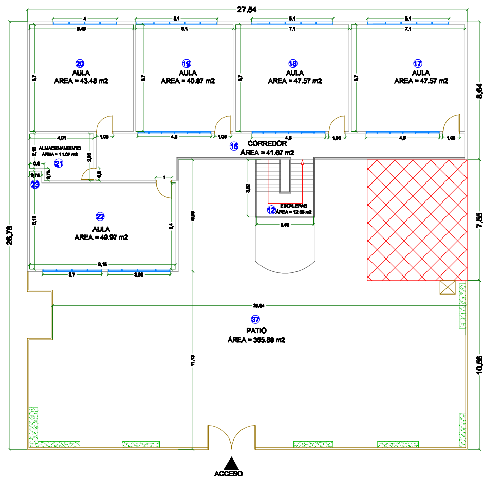
PLANTA SEGUNDO PISO
