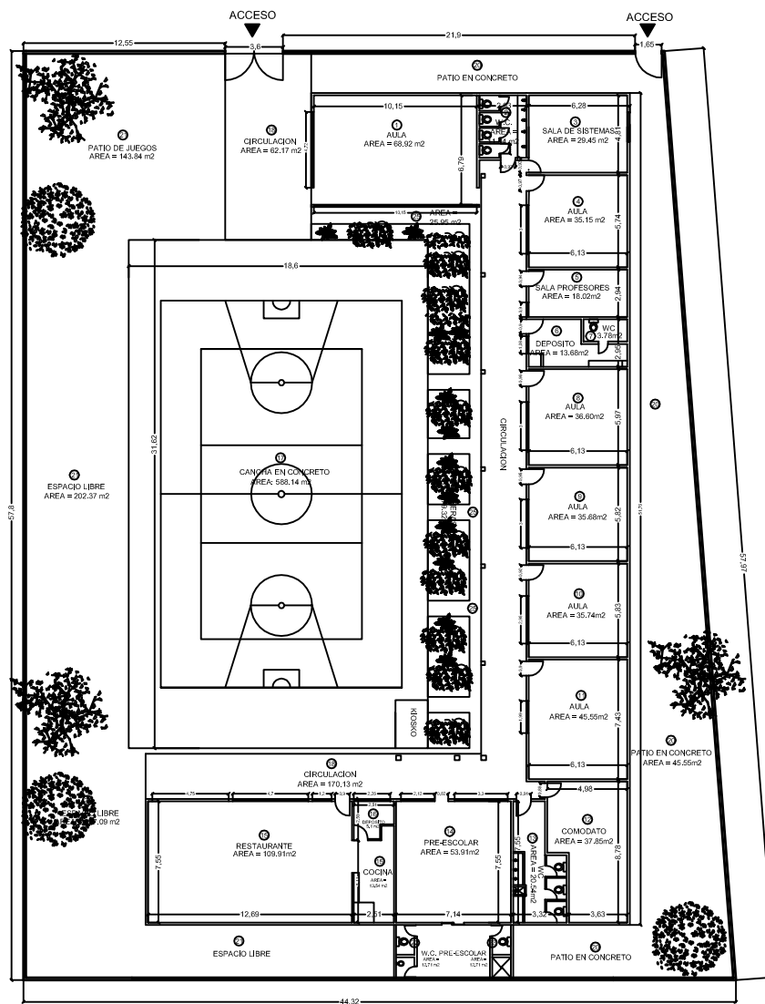
PLANTA PRIMER PISO
