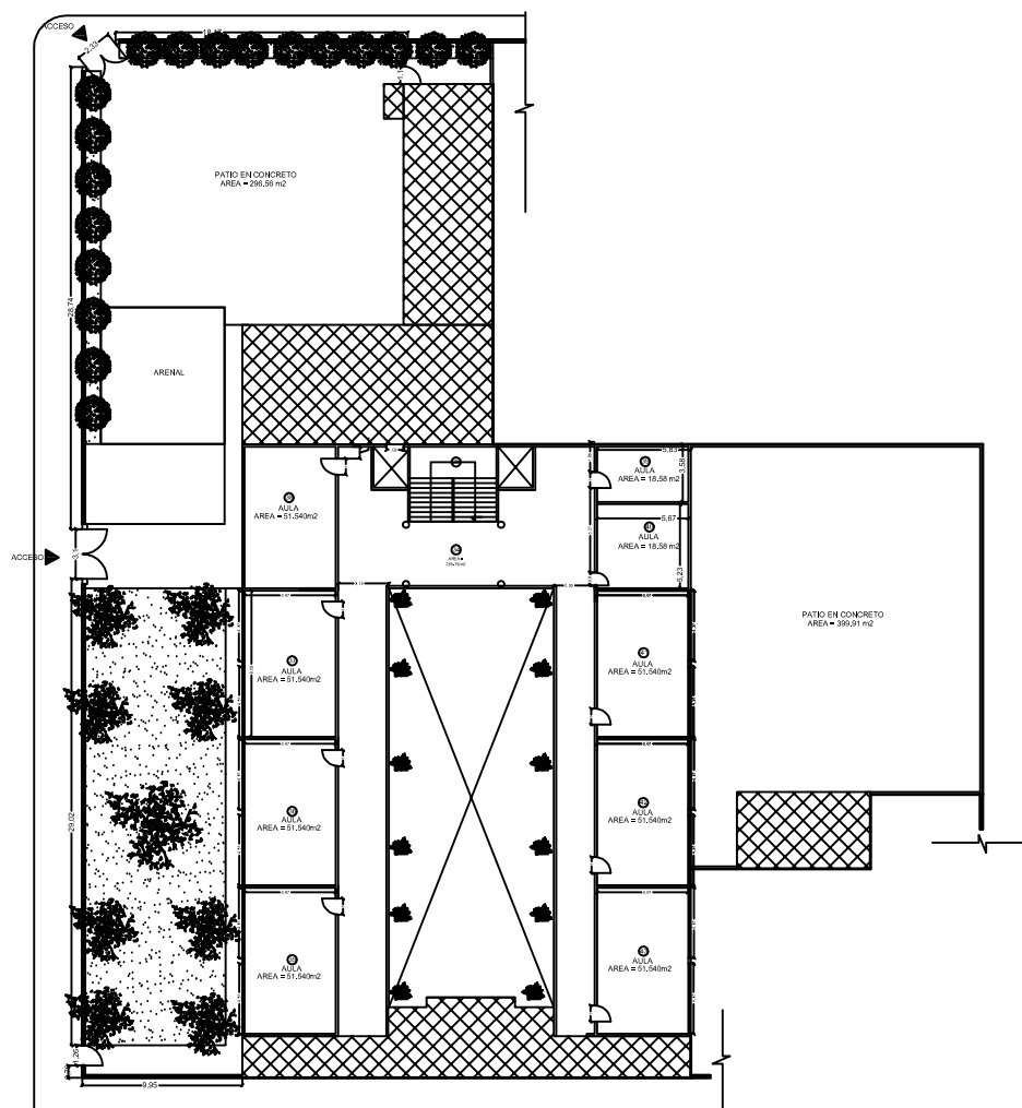
PLANTA SEGUNDO PISO
