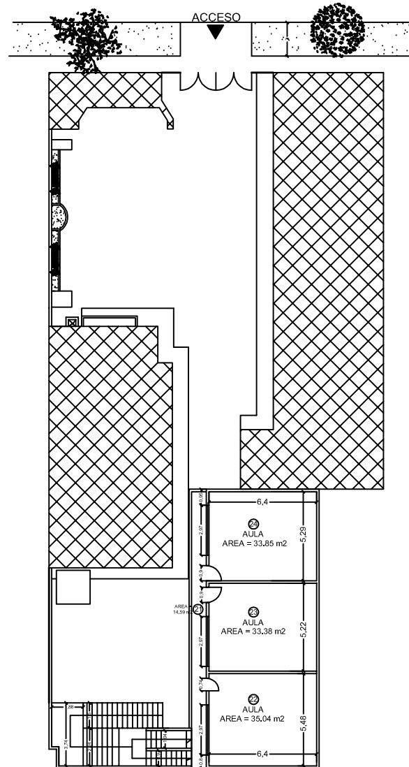
PLANTA TERCER PISO
