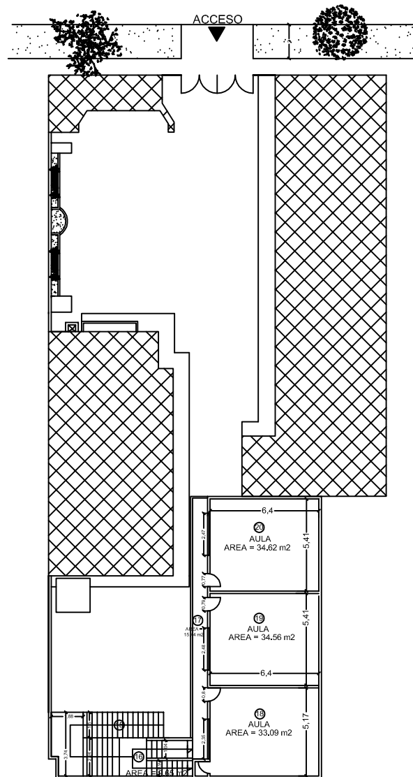
PLANTA SEGUNDO PISO
