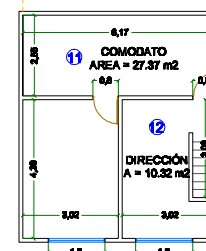
PLANTA SEGUNDO PISO
