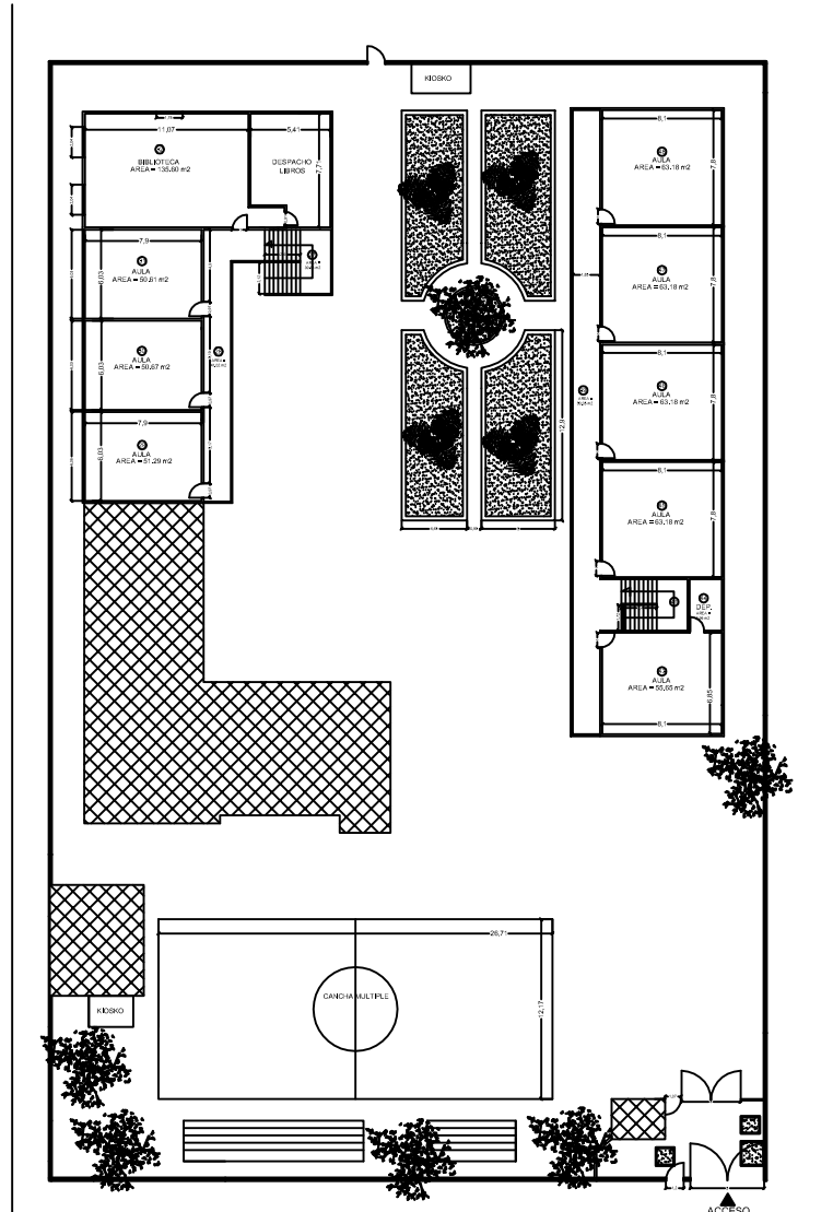
PLANTA SEGUNDO PISO
