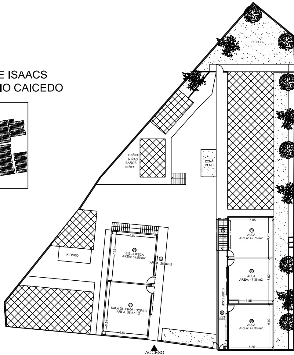
PLANTA SEGUNDO PISO
