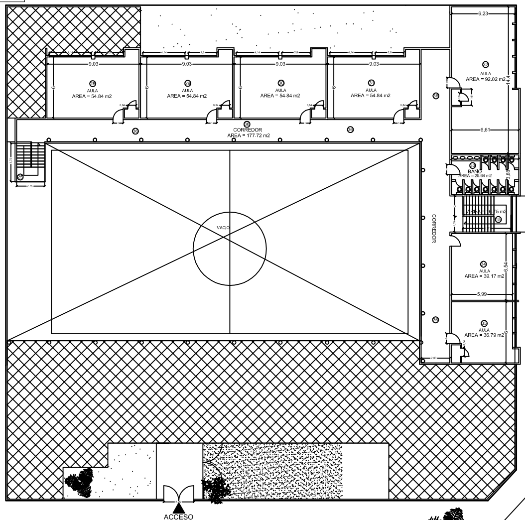
PLANTA SEGUNDO PISO
