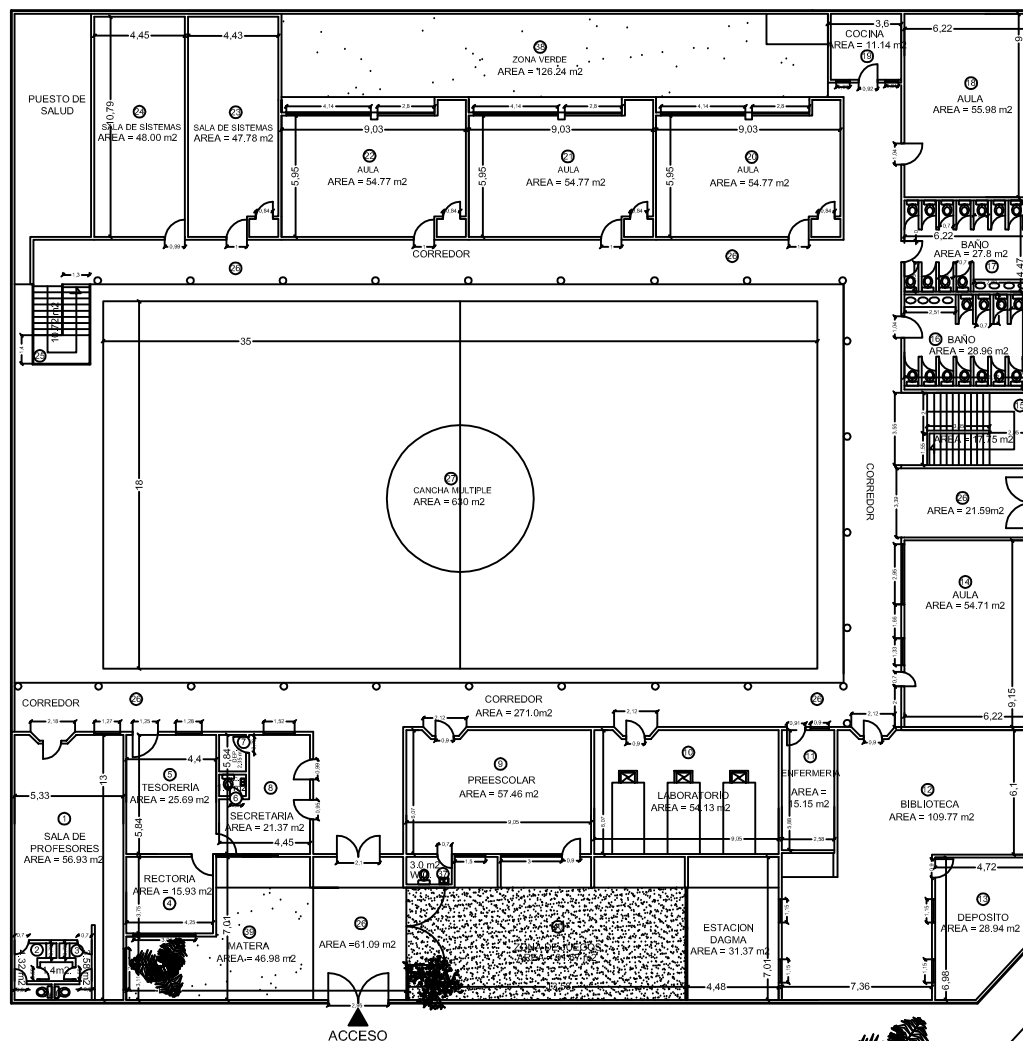
PLANTA PRIMER PISO
