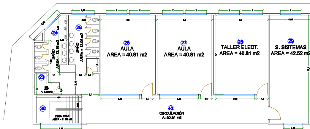
PLANTA SEGUNDO PISO
