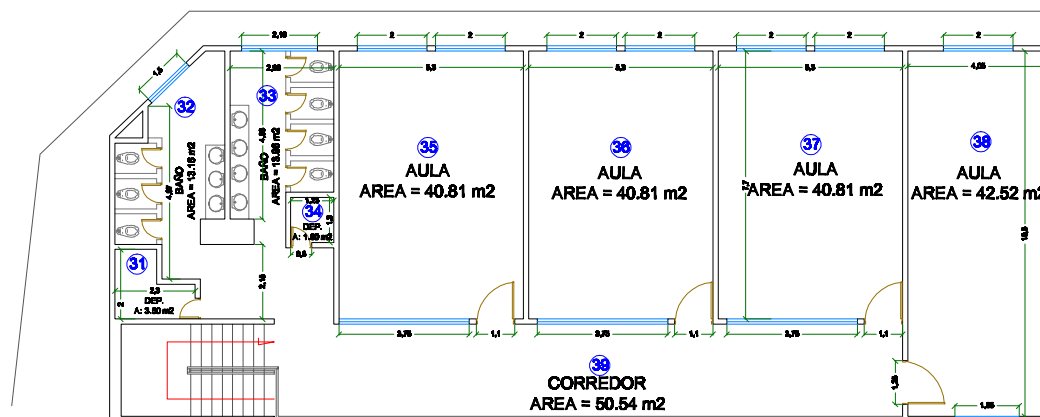
PLANTA TERCER PISO
