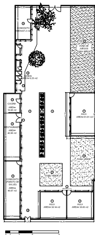
PLANTA PRIMER PISO
