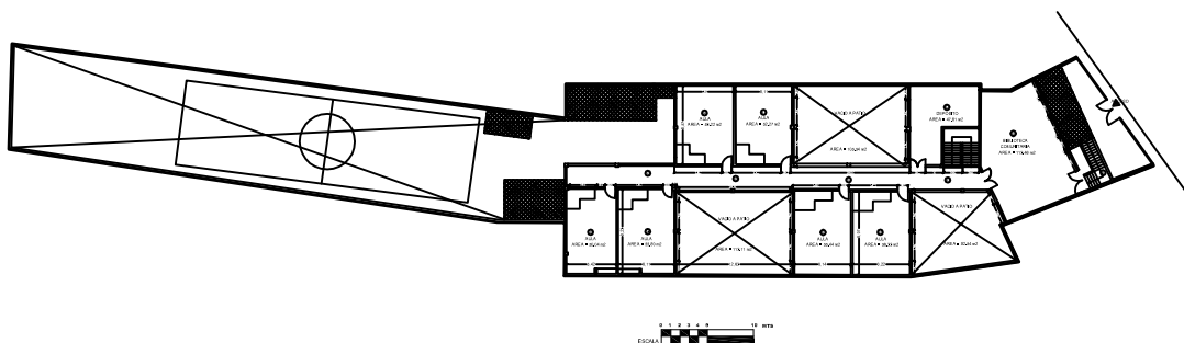
PLANTA SEGUNDO PISO
