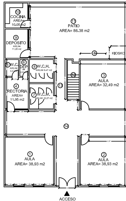
PLANTA PRIMER PISO
