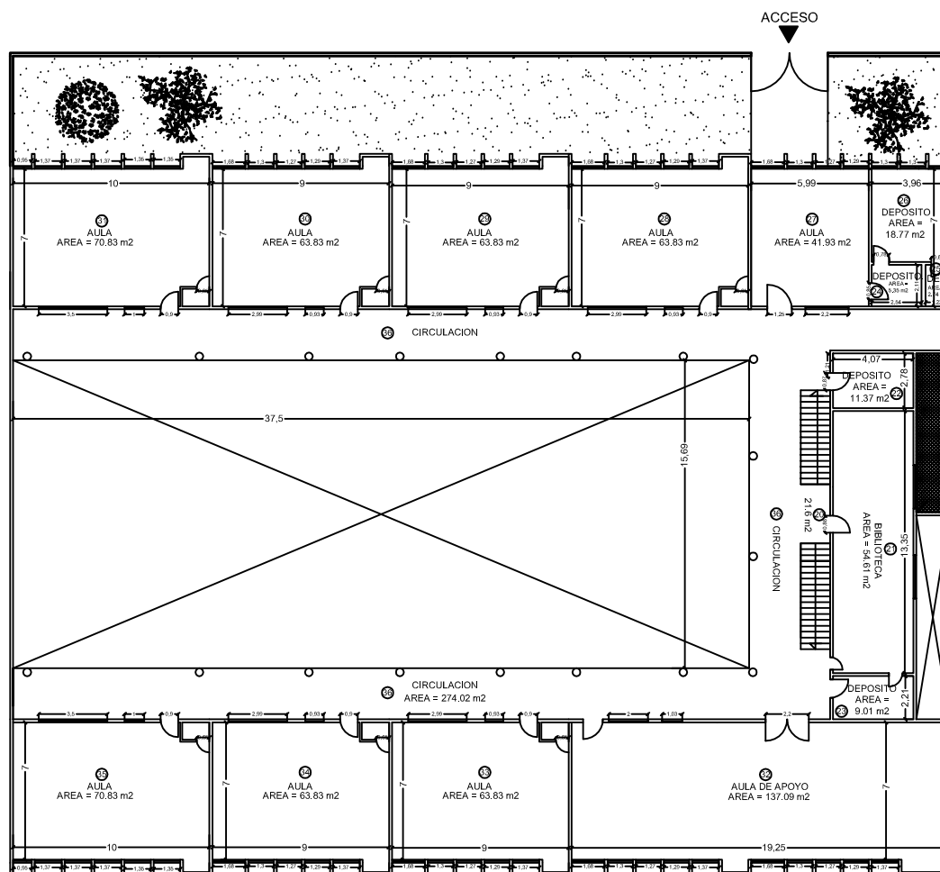
PLANTA SEGUNDO PISO
