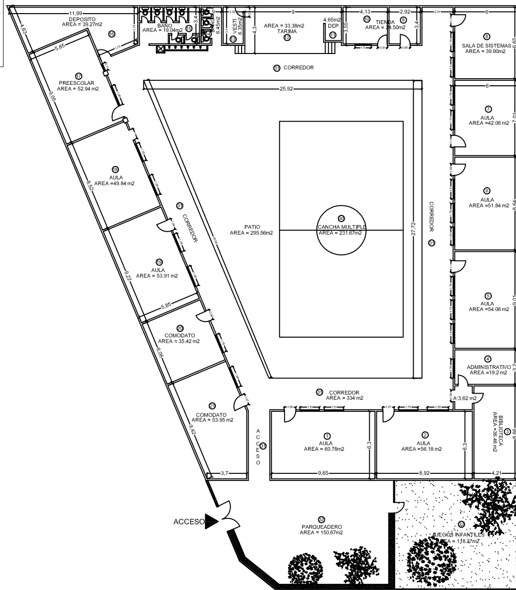
PLANTA PRIMER PISO
