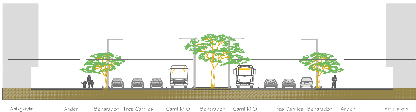
PERFILES SISTEMA DE TRANSPORTE MASIVO MIO SEGUN MECEP
