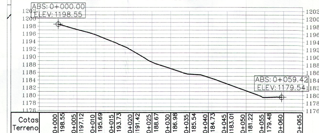
Perfil Longitudinal: PERFIL 3 Escala - V: 500 H:500
