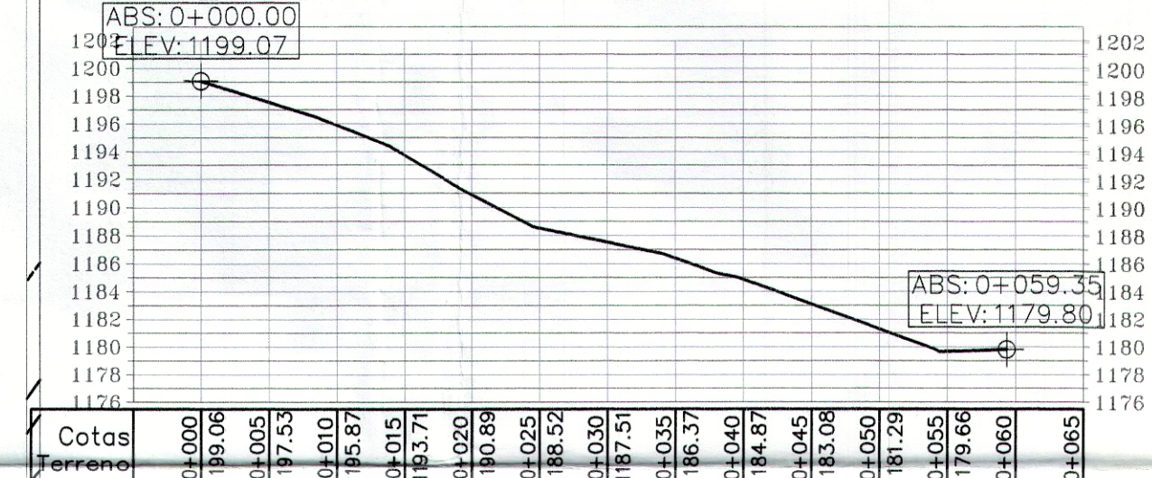
Perfil Longitudinal: PERFIL 2 Escala - V: 500 H:500
